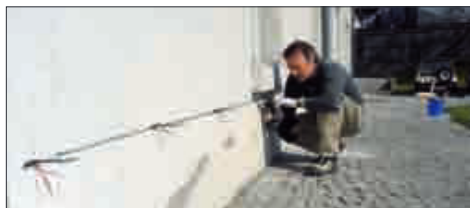
Bilgeri-Kaserne, Bregenz; Einlegen der Wandelektroden infolge aufsteigender Feuchtigkeit.
